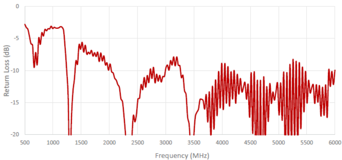
Cable 1: 5GNR
