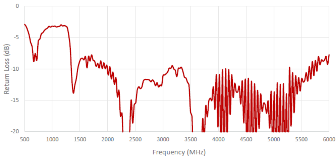
Cable 3: 5GNR
