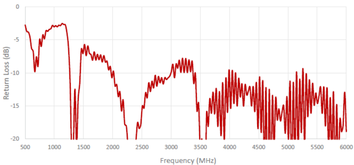
Cable 2: 5GNR
